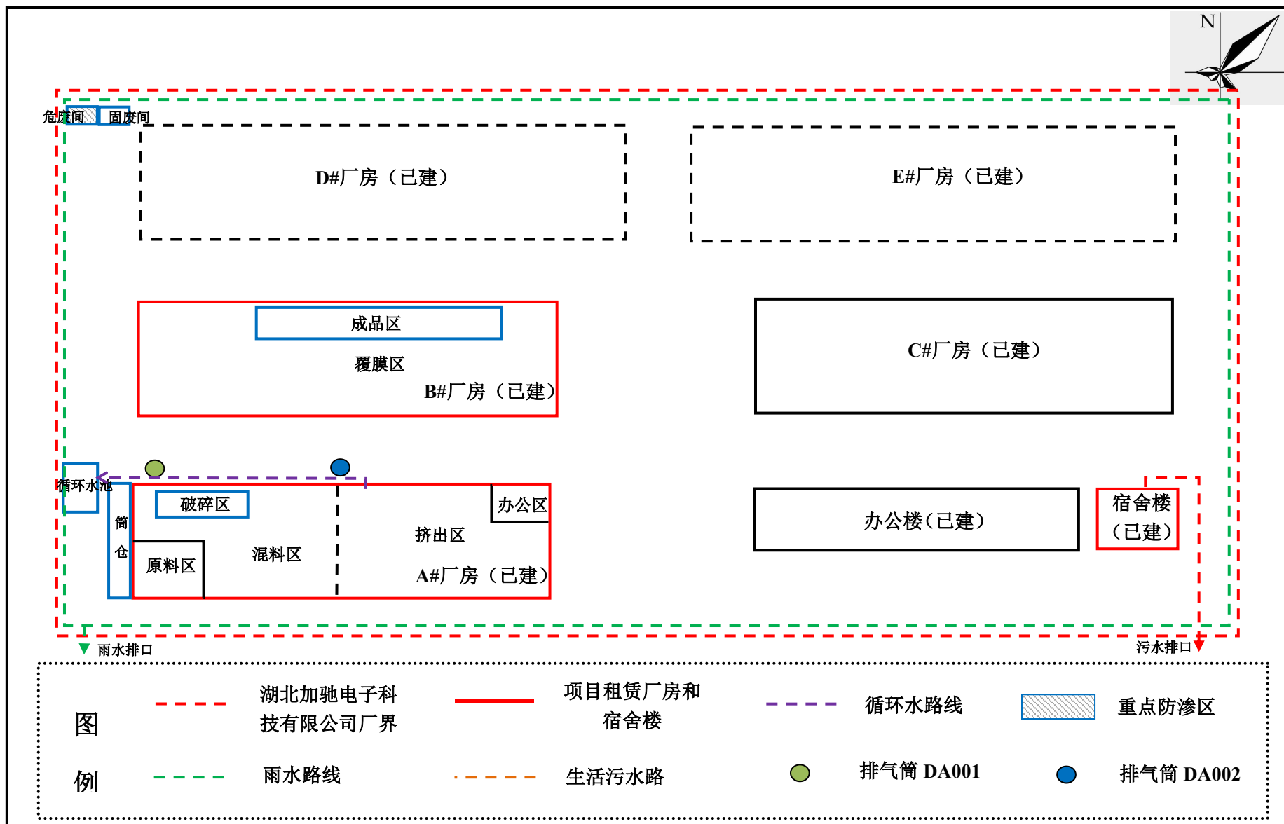
附图3 项目厂区平面布局图及雨污管网图
