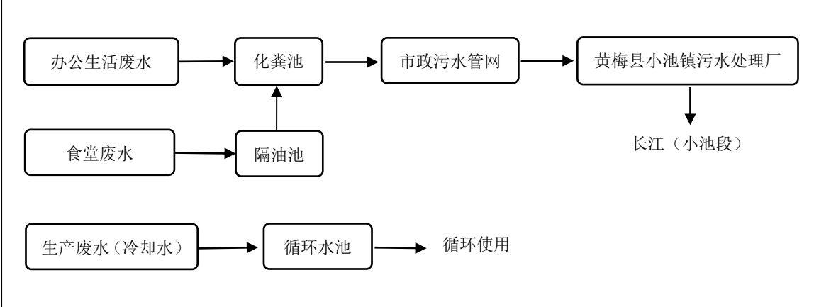
图 3-4 项目废水处理工艺流程图
