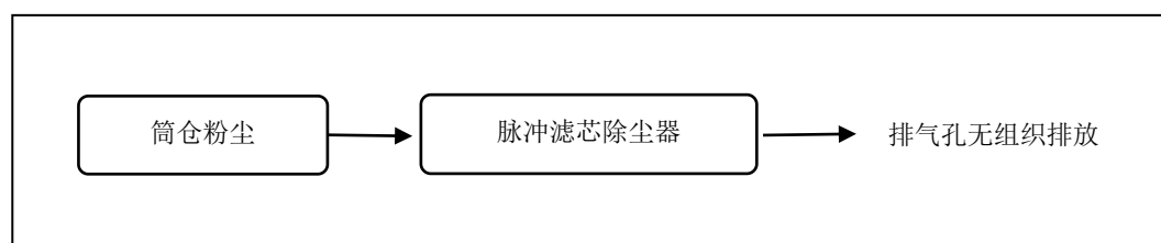
图 3-3 项目筒仓粉尘处理工艺流程图
