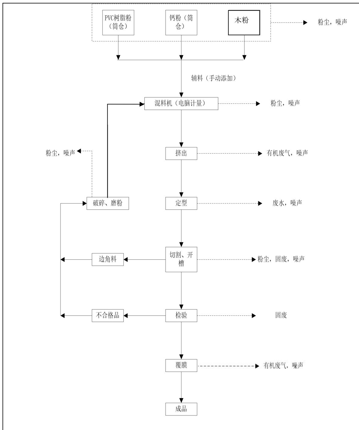
图 2-3 项目生产工艺流程及产污节点图
