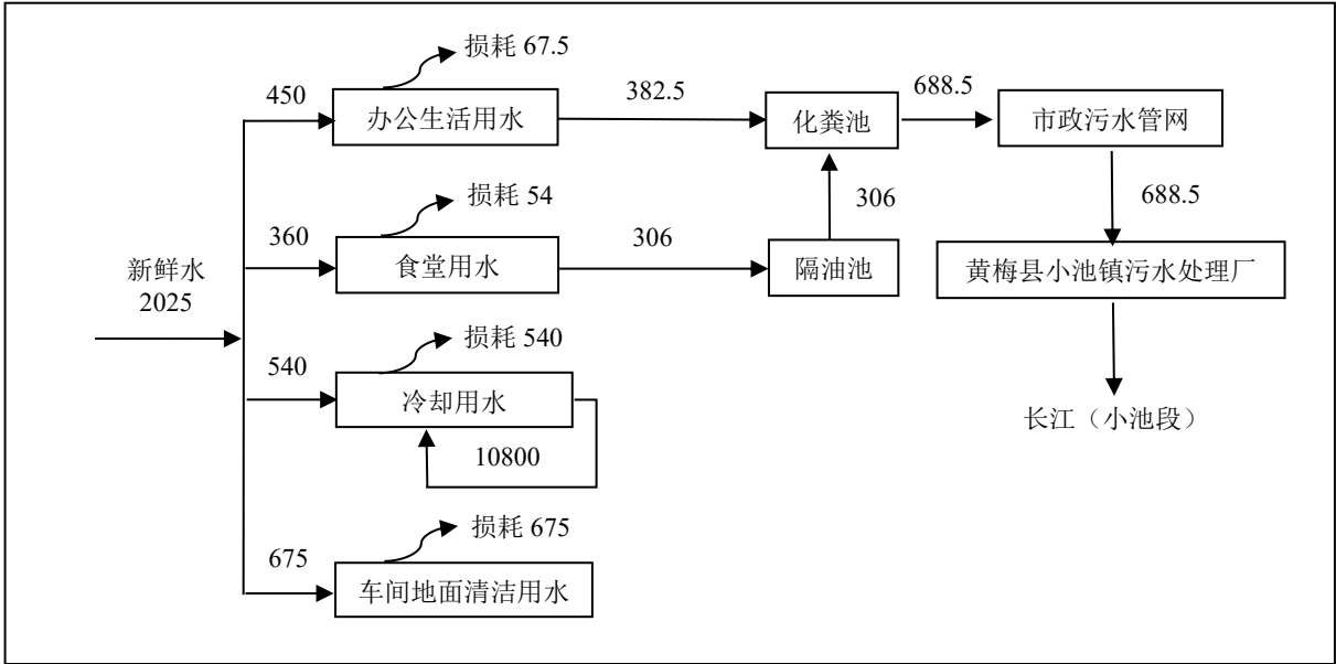
图 2-2 项目水平衡图（单位：m 3 /a）
