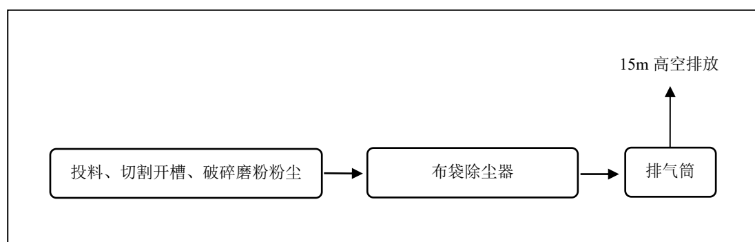
图 3-1 项目投料、切割开槽、破碎磨粉粉尘处理工艺流程图
