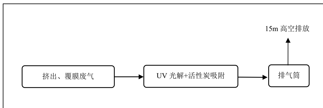
图 3-2 项目挤出、覆膜废气处理工艺流程图
